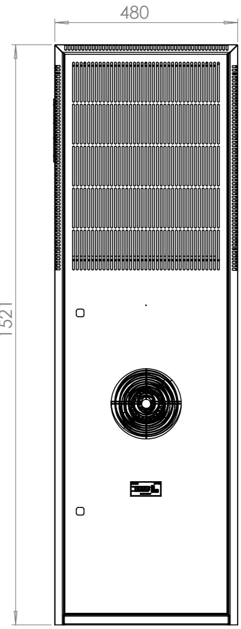
ÖN GÖRÜNÜŞ
