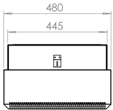
ÜST GÖRÜNÜŞ
